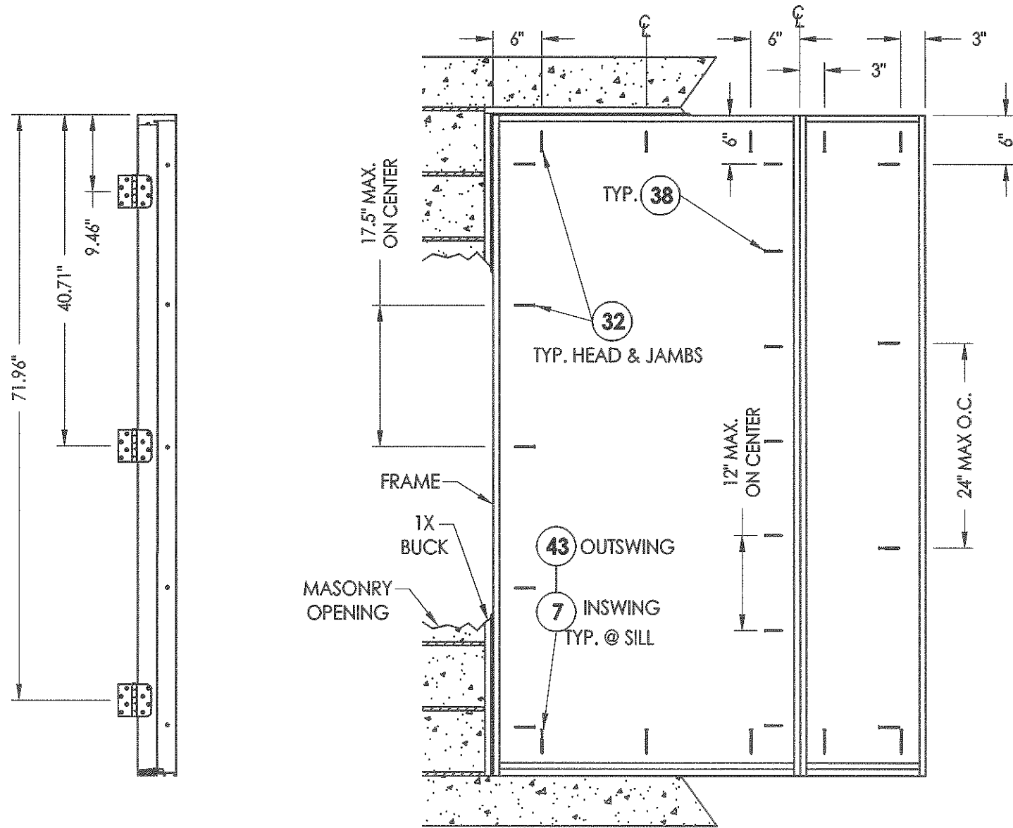
HINGE JAMB
